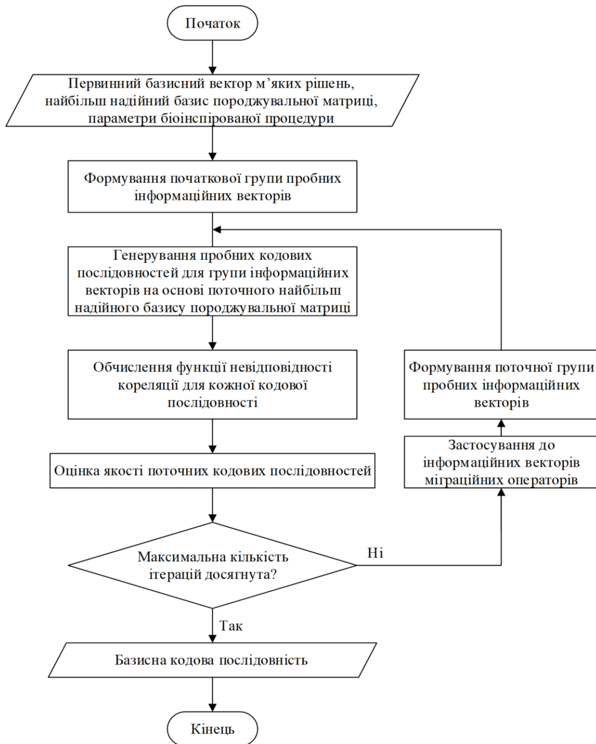
Рис. 3. Схема алгоритму підпроцесу біоінспірованого пошуку кодового слова алгебраїчних згорткових кодів
