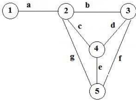
Рис. 2. Граф сети
