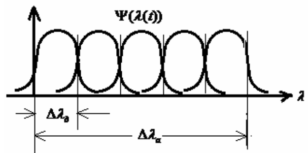
Рис. 3. Характеристика багатоканального вимірювача параметра \lambda
