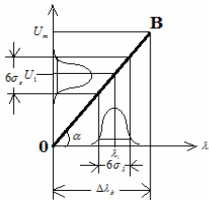
Рис. 1. Характеристика ОВ – шкала вимірювача: 6\sigma_3 – довірчий інтервал завади з квантилем рівним 3; 6\sigma_\lambda – довірчий інтервал параметра з квантилем рівним 3; U_m, U_1, \lambda_1, \Delta\lambda_0 – відповідно максимальна напруга на межі діапазону відліків, відлік, точкова оцінка параметра та апертура, або діапазон вимірювача
