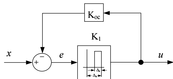
Рис. 2. Структурна схема системи формування ЧІМ-закону керування з двопозиційною характеристикою
