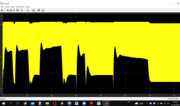
Рис. 10. Графік зміни коефіцієнта K_{Понт} за наявності завад змінної інтенсивності
