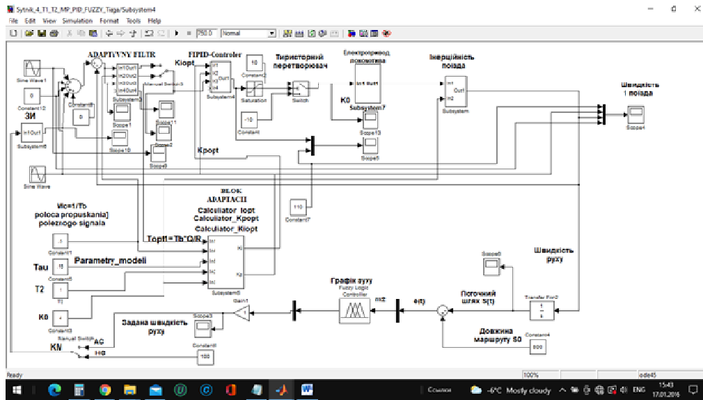
Рис. 5. Структурна схема моделі контуру керування, що включає регулятор, адаптивний фільтр, блок адаптації коефіцієнтів налаштування регулятора і блок моделі нечіткого задавання графіка прямивання
