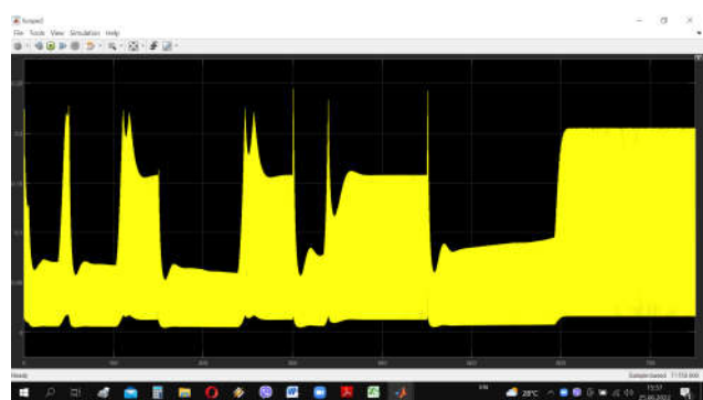
Рис. 20. Графік зміни оптимальної постійної часу адаптивного фільтра T_{opt}(Q, R, T_0) за наявності завод змінної інтенсивності
