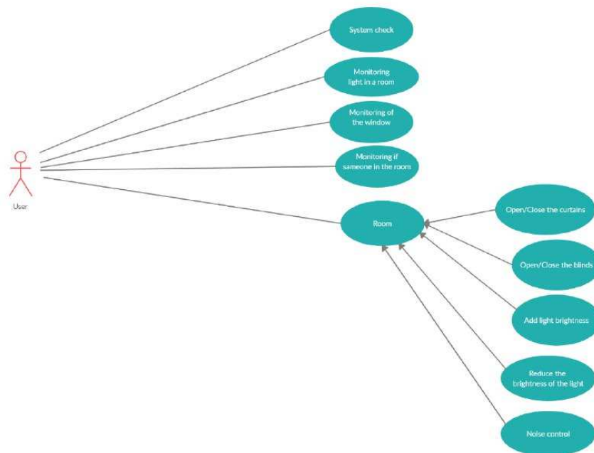
Рис. 4. UML діаграми-використання
